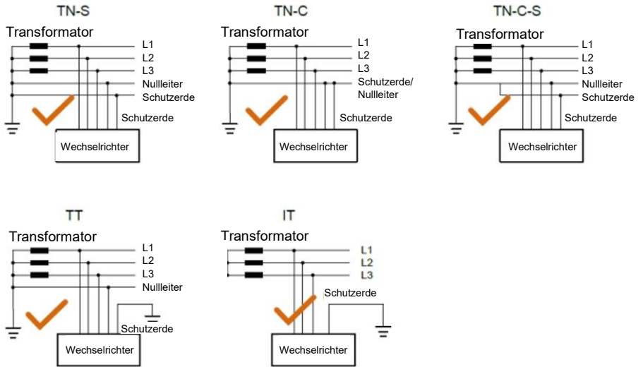
Abb. 2.2 Netzformen, die von netzgebundenen PV-Wechselrichtern unterstützt werden
