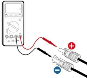
Abb. 5.4 Eingangsspannung messen
