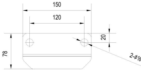
Abb. 4.7 Abmessungen Montagewinkel
