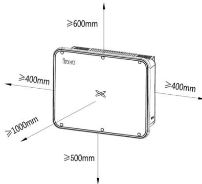
Abb. 4.4 Installationsabstände
