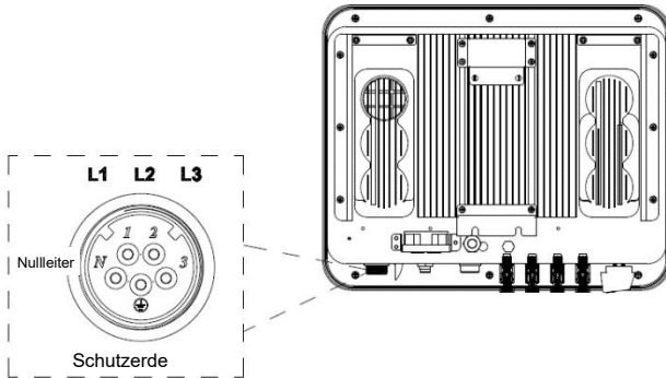
Abb. 5.9 Netzanschluss des dreiphasigen Wechselrichters
