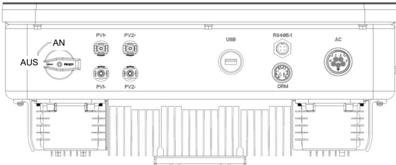
Abbildung 2.10 XG3-12KTR Unteransicht
