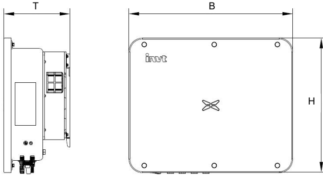
Abbildung 2.5 Abmessungen des Wechselrichters
