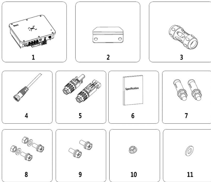
Abb. 4.1 Lieferumfang eines dreiphasigen Wechselrichters 3 - 15 kW
