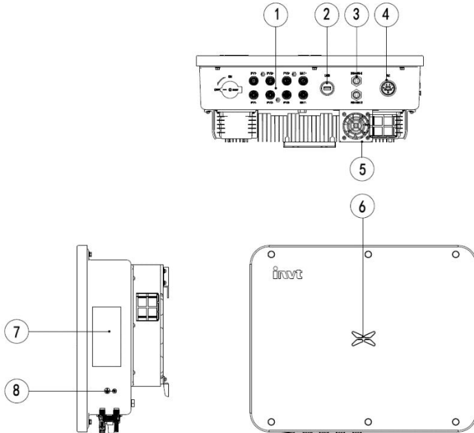
Abbildung 2.3 Erscheinungsbild des dreiphasigen PV-Wechselrichters
