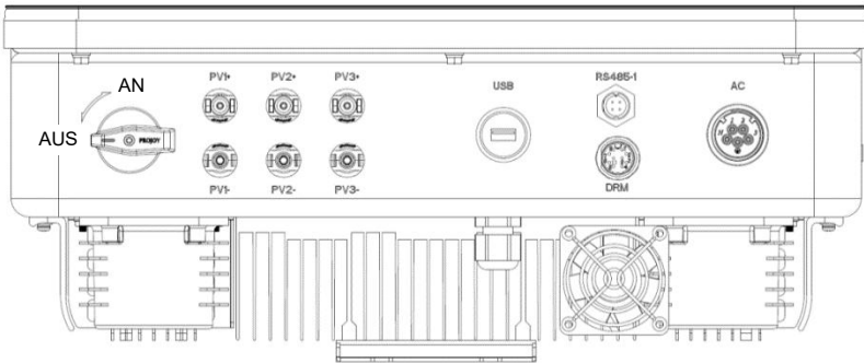
Abbildung 2.9 XG15KTR1 Unteransicht
