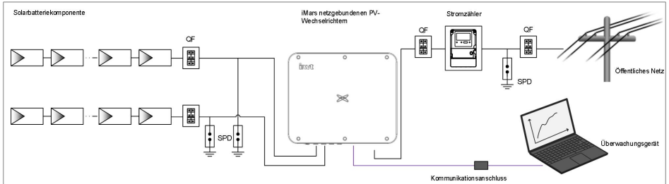
Abb. 5.1 Schematische Darstellung des Anschlusses einer netzgebundenen PV-Anlage
