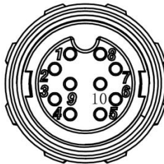
Abb. 5.7 DRM- und RS485-Anschluss Draufsicht
