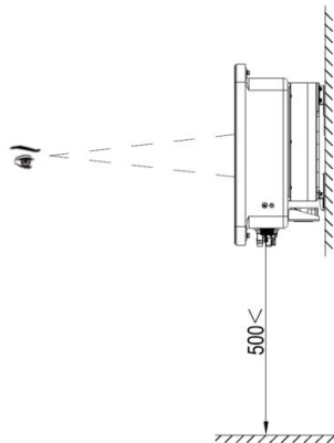
Abb. 4.3 Optimale Installationshöhe
