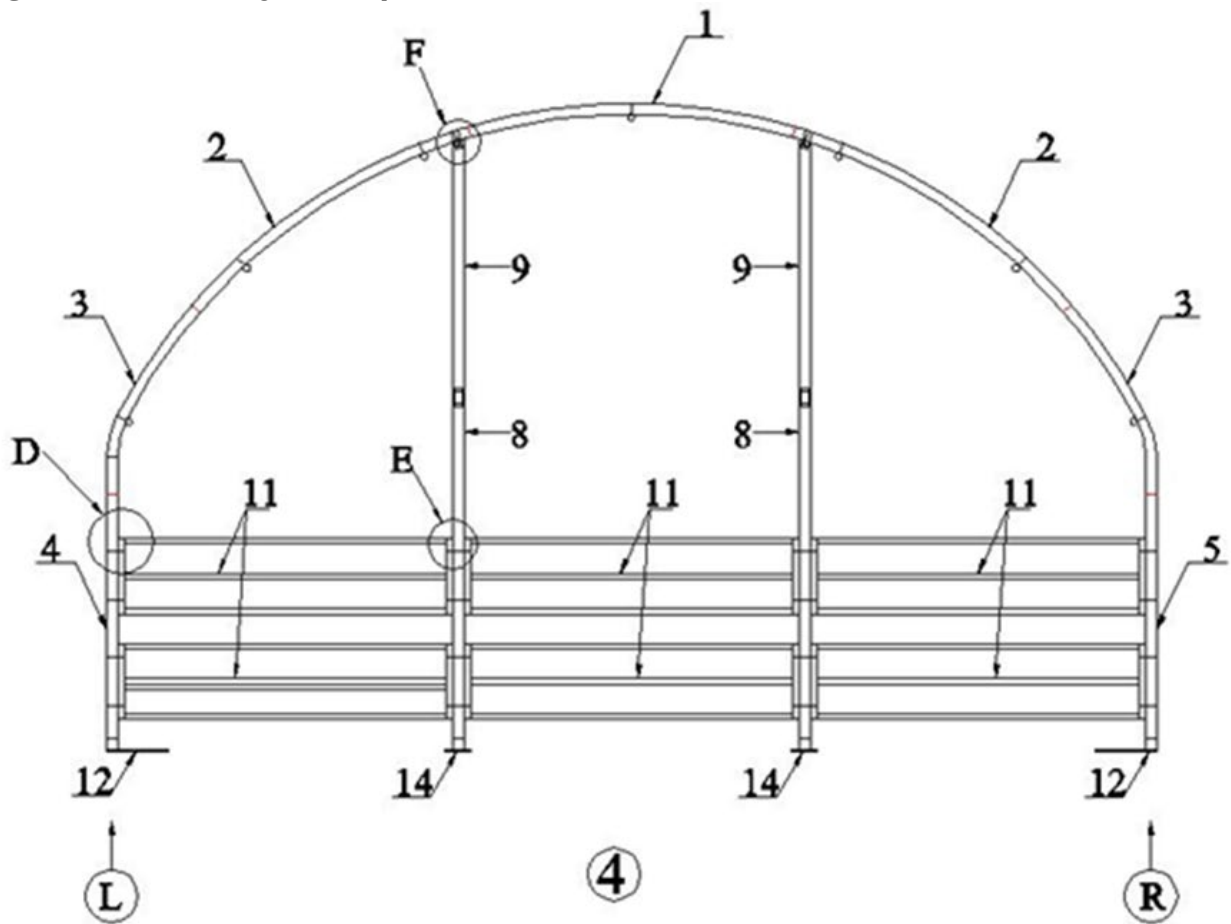
Fig 4: Den sista böjen (4), portaler och staket
