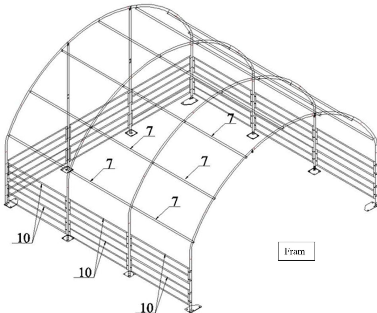
Fig 6: Uppsättning av ställning, säkring av stolpfötter med pålpinnar
