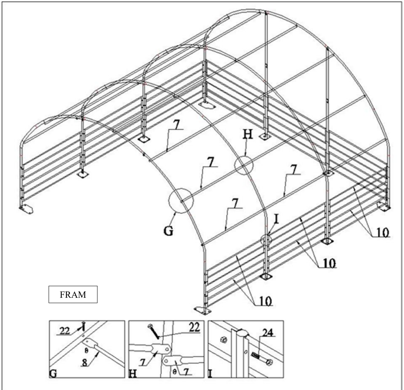
Fig 5: Läkt och sidoväggar
