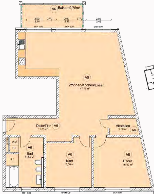
Haus A Wohnung A6
