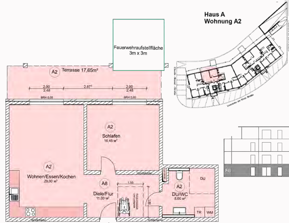
ERDGESCHOSS HAUS A WE A2
