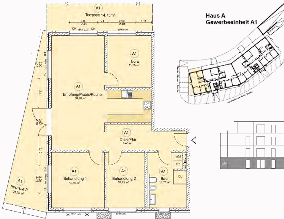
ERDGESCHOSS HAUS A WE A1
