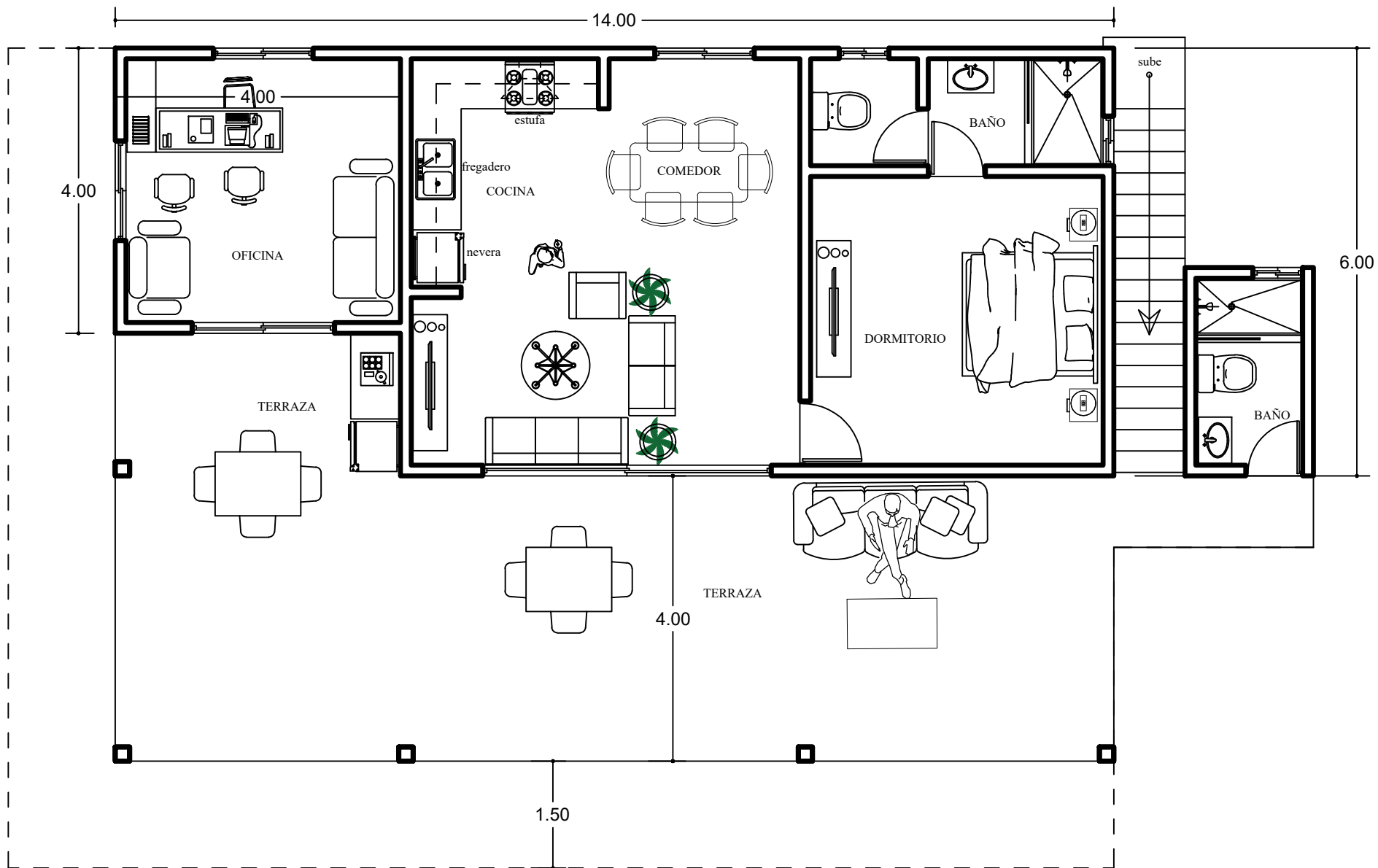
1er nivel casa 60 mt2
