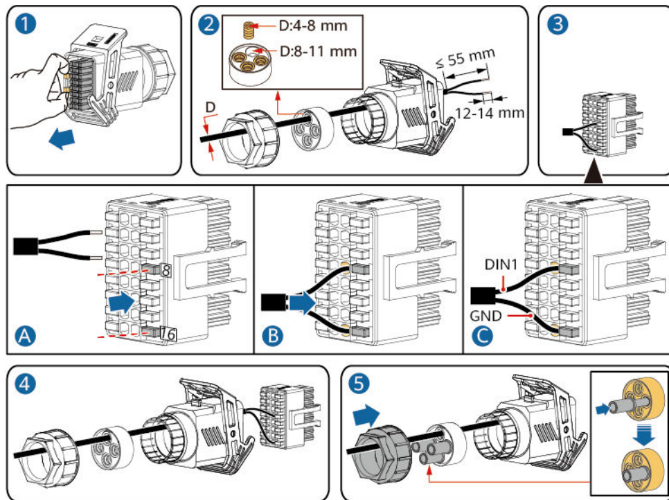
Abbildung 5-36 Kabelmontage
